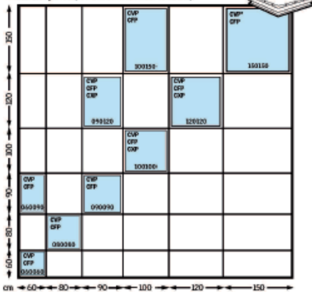
Finestra capoline (dimensioni del foro nel solaio)
